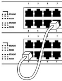
Abbildung 1-4. Kaskadieren von Switches
